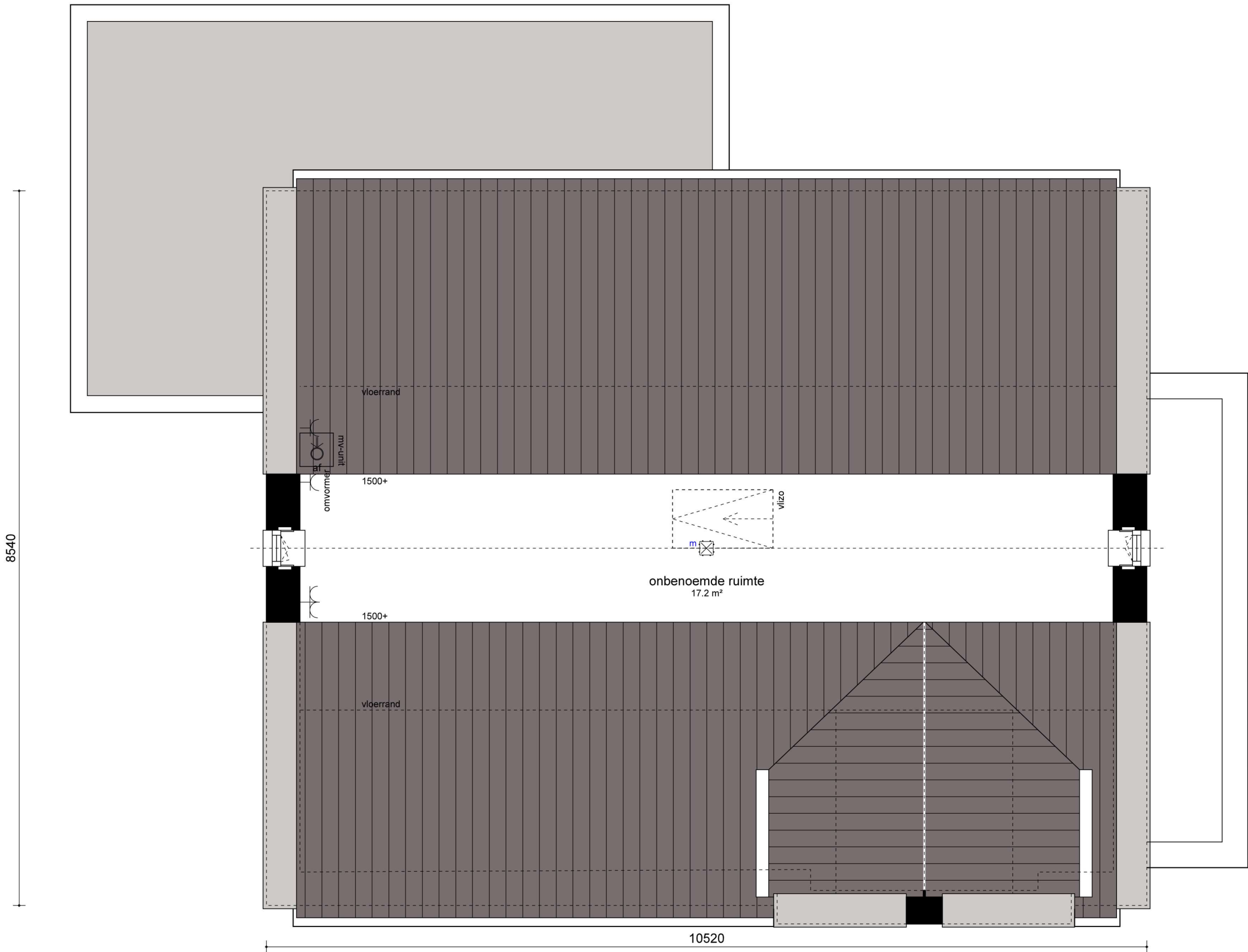
SCHAAL 1 OP 50 Plattegrond ~ Tweede verdieping
